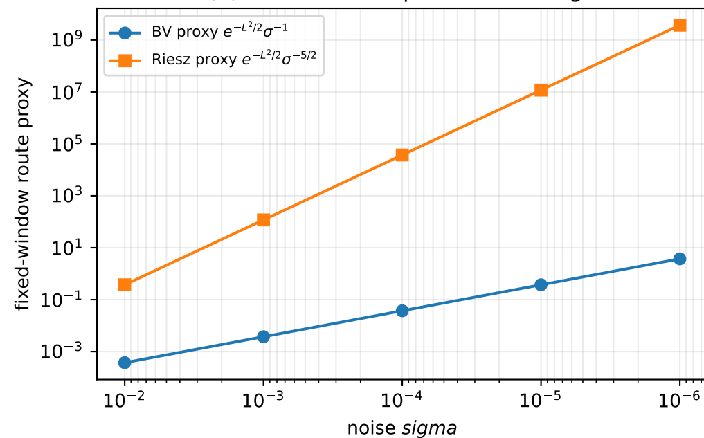
(d) Fixed-window proof-route no-go
