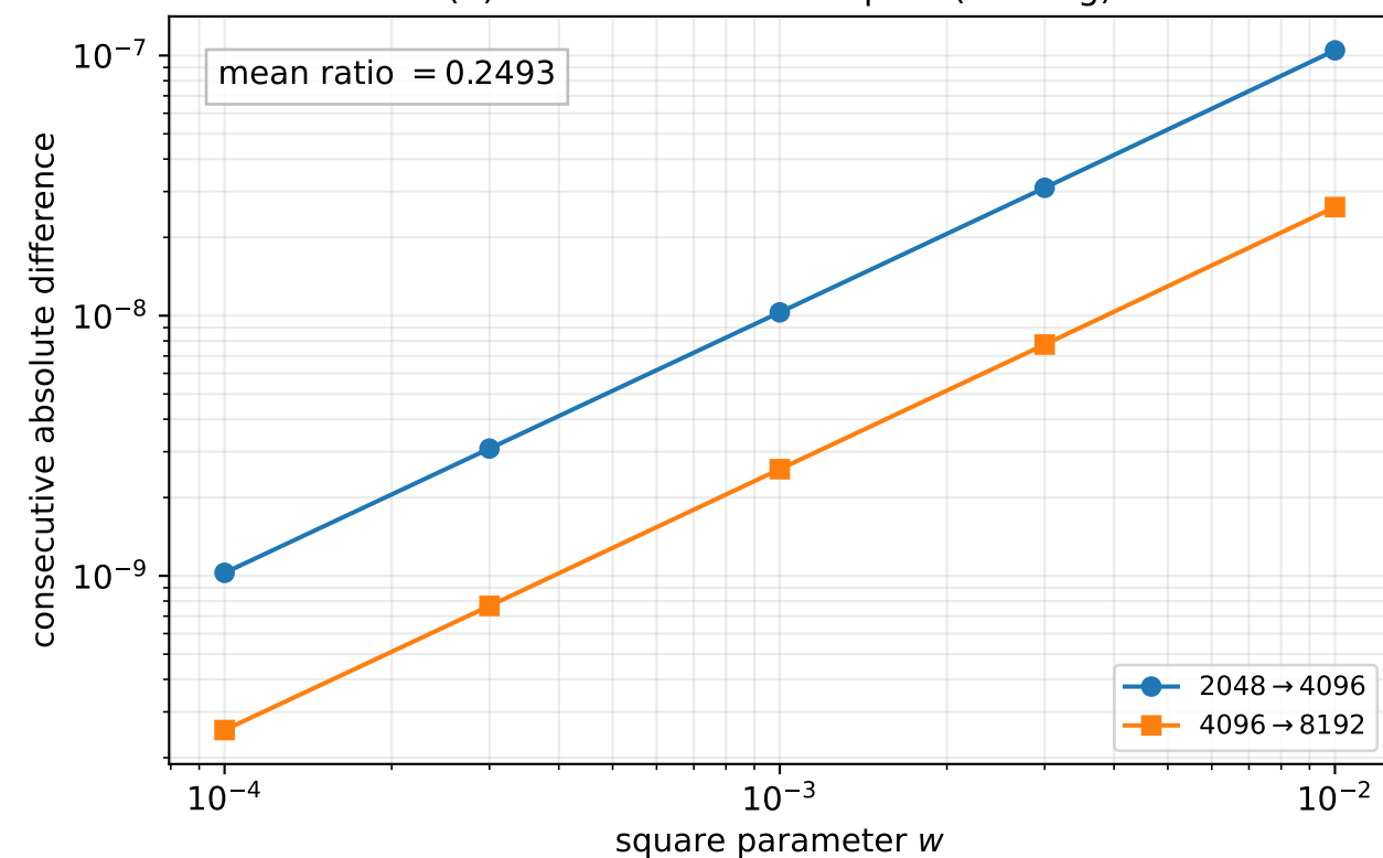
(d) Stored determinant pilot (floating)
