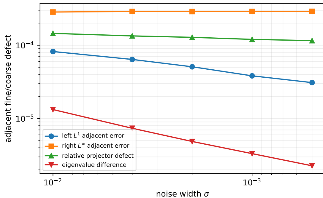
(d) Intrinsic factors are stable across one Haar level
