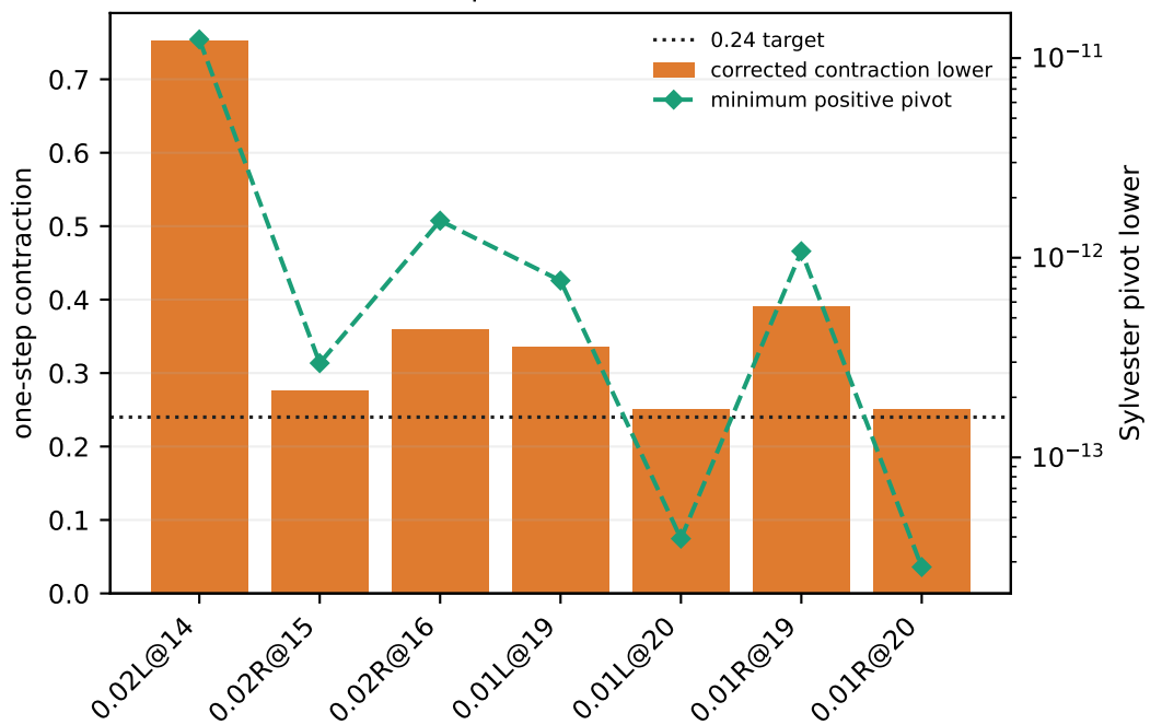
(d) Seven pointwise obstructions
