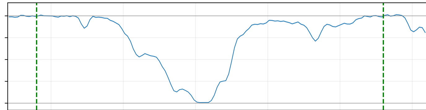
Fe II 1608
