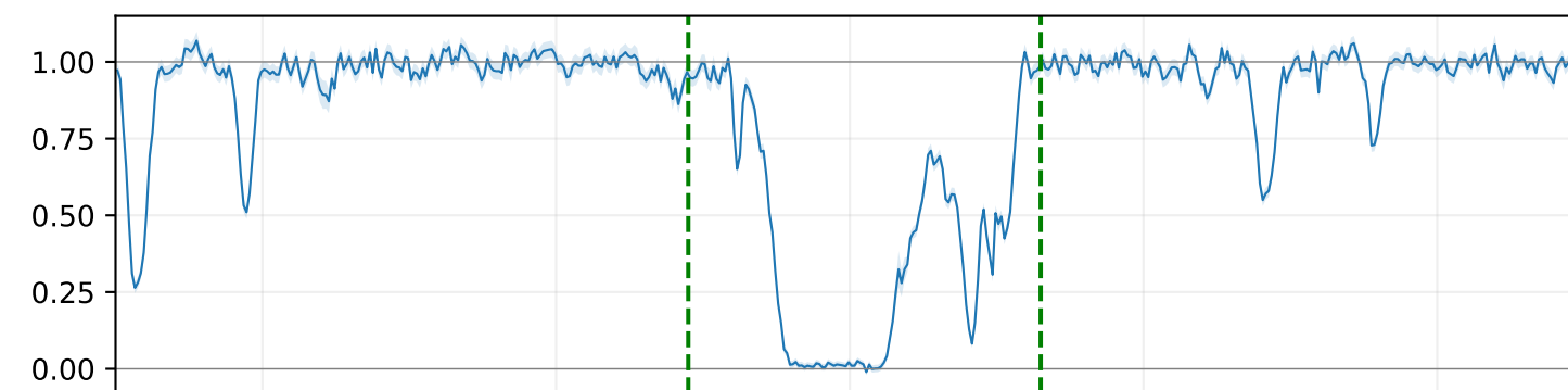
Fe II 2382
