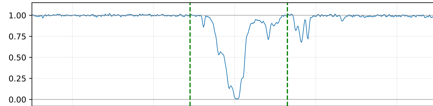
Fe II 1608
