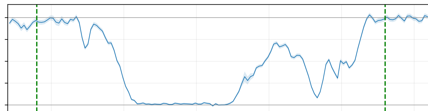
Fe II 2382
