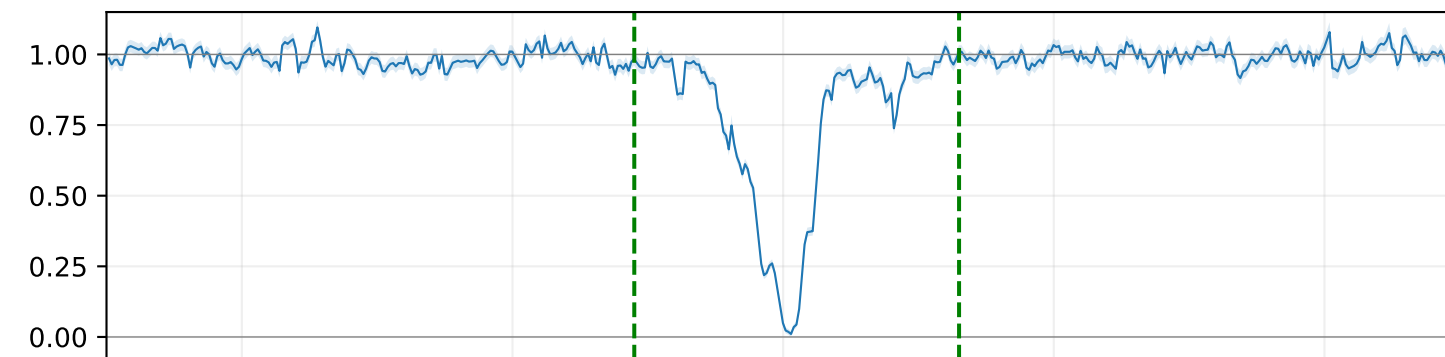
Fe II 2374
