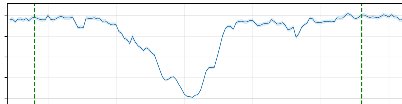
Fe II 2374
