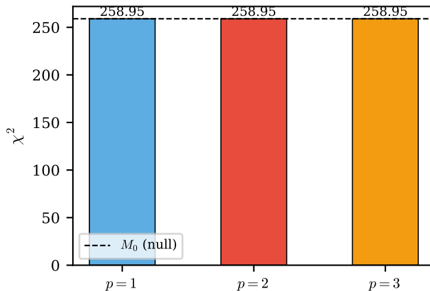
(d) \chi^2 comparison: 1/\ln^p models
