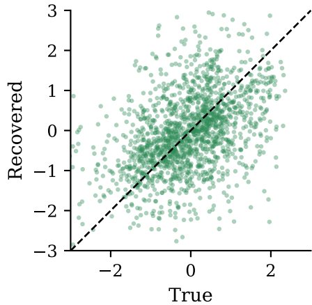
(d) 2D+3D: Test (S) r = 0.414
