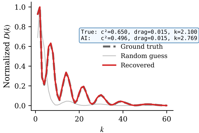
(b) Parameter recovery
