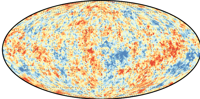
(a) Planck SMICA (Nside=32)
