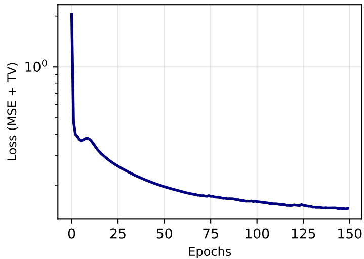
(d) Convergence ( r=0.929 )
