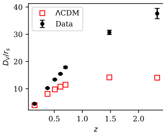
(e) BAO
