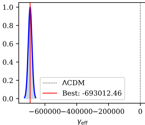
(d) CMB TT residual
