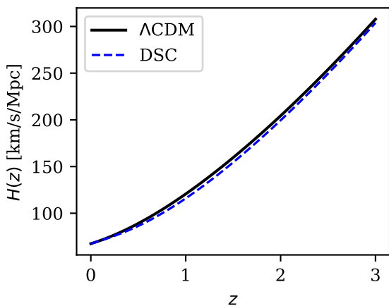
(e) BAO
