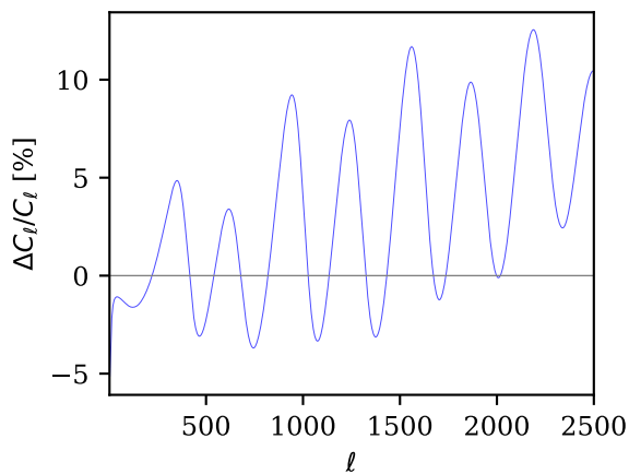
(d) CMB TT residual
