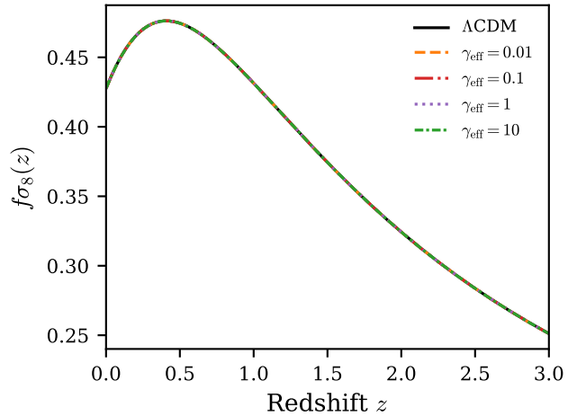
(d) Growth rate f\sigma_8
