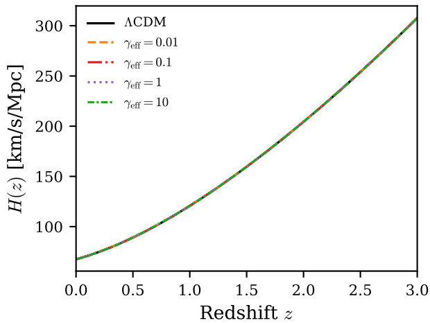
(a) Hubble parameter H(z)
