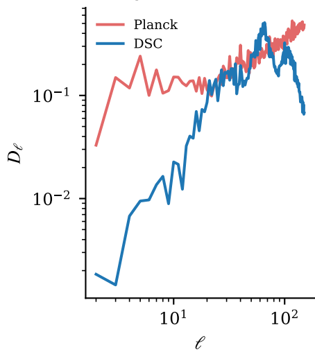
(d) Angular power spectrum
