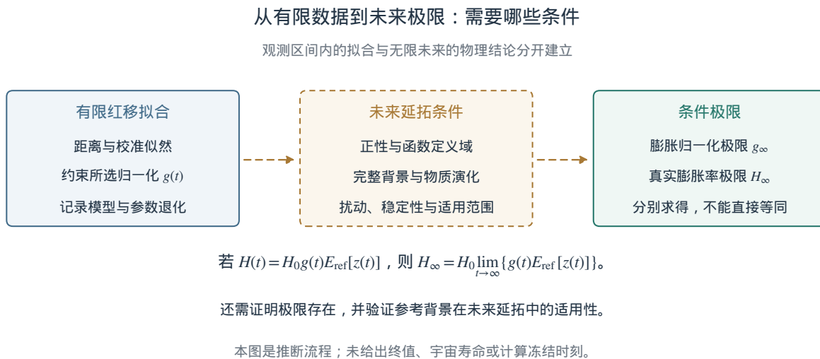
图5.3 未来外推的物理接口。 有限红移范围的拟合、响应正性、完整背景及扰动检验分别承担不同任务。函数极限可作为条件研究对象, 确定的宇宙终局仍须由完整模型给出。
