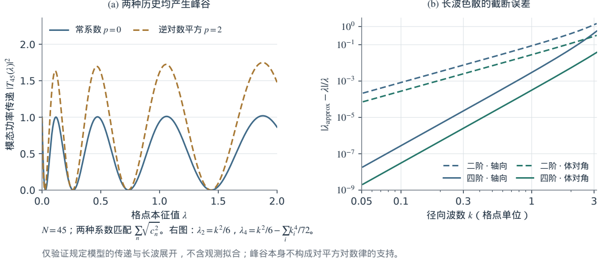
图4.2 微观迭代的可计算宏观读数。左图比较 N = 45, c_0 = 10, A_2 = 0.45 的逆对数平方历史与常数历史；后者匹配相同 s_N ，两者均产生振荡传递。右图比较六邻域精确本征值与长波展开，分别沿坐标轴及空间对角方向显示二阶、含四阶修正的相对误差。曲线由独立验证脚本生成，不使用天空数据，也不比较观测拟合优劣。 53
