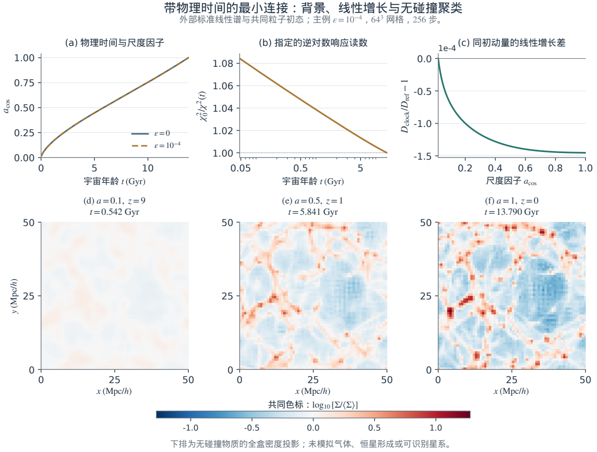
图4.4 从物理背景到无碰撞物质聚类。 上排为尺度因子与年龄、时钟归一化响应 \chi_0^2/\chi^2 及相同初动量下的线性增长差；下排为主例在 z = 9, 1, 0 的实际存档密度投影，使用共同对数色标。标准引力及外部CAMB初谱是本轮的物理输入，两背景共享同一初态。主格距 0.78125 \text{ Mpc}/h 、每粒子质量 4.17 \times 10^{10} M_\odot/h ；本图展示物质聚类，未分辨星系。功率图、各分辨率结果及核验见实验归档。 57
