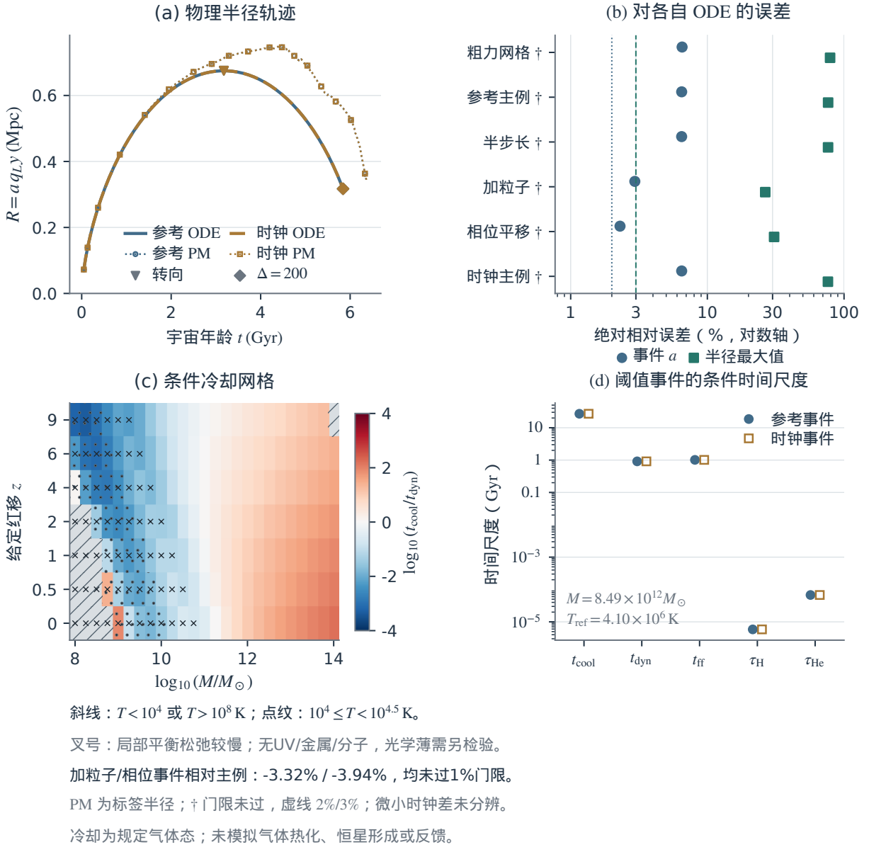
图4.5 受控塌缩与气体冷却接口的结果及边界。 左上比较连续球形方程与主PM的半径一年龄轨迹，PM使用固定标签的中位半径代理；右上保留全部六配置的事件和共同事件前半半径误差，2%与3%虚线是协议中针对主配置的精度要求，其他配置按各自条款检查。左下为175个唯一质量-红移状态的瞬时冷却/动力学时间比，两背景在相同状态下共用读数；灰色斜线表示 T < 10^4 K或 T > 10^8 K，点纹标记 10^4 - 10^{4.5} K敏感区，叉号表示局部电离平衡警示。右下只使用两个经过独立核验的连续球形事件，未将失败的PM代理作为气体密度或温度输入。标准引力、原初气体速率和特征气体状态均为本轮规定的物理条件。 62
