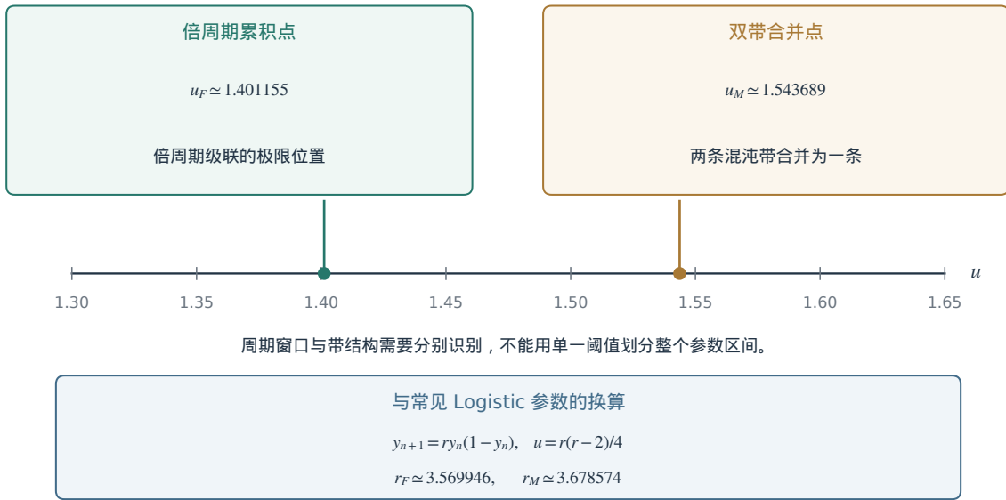
图2.2 固定参数二次族的两个不同事件。 图中区分倍周期积聚点与双带合并点，并列出logistic坐标下的对应参数。横向位置是参数示意，不是本轮计算的分岔图；未将整段参数区间划为单一动力学状态。数值与坐标约定见式(2.4)及文献27、28。
