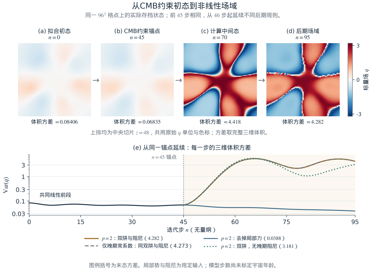
图4.3 从数值初态到后期结构的演化时间线。 上排为 n = 0, 45, 70, 95 的真实中央切片，使用相同的有符号场色标；下排为完整三维体积的逐步方差及对照。全部分支共享前45步的历史及两态锚点；“仅晚期常系数”只替换第46—95步的系数。第45步后的局部势和阻尼按已记录方案给定。初态受同一CMB拟合约束，末态为标量场域，两者尚未分别识别为真实大爆炸初态与星系。图由既有结果的小型来源快照重绘。24
