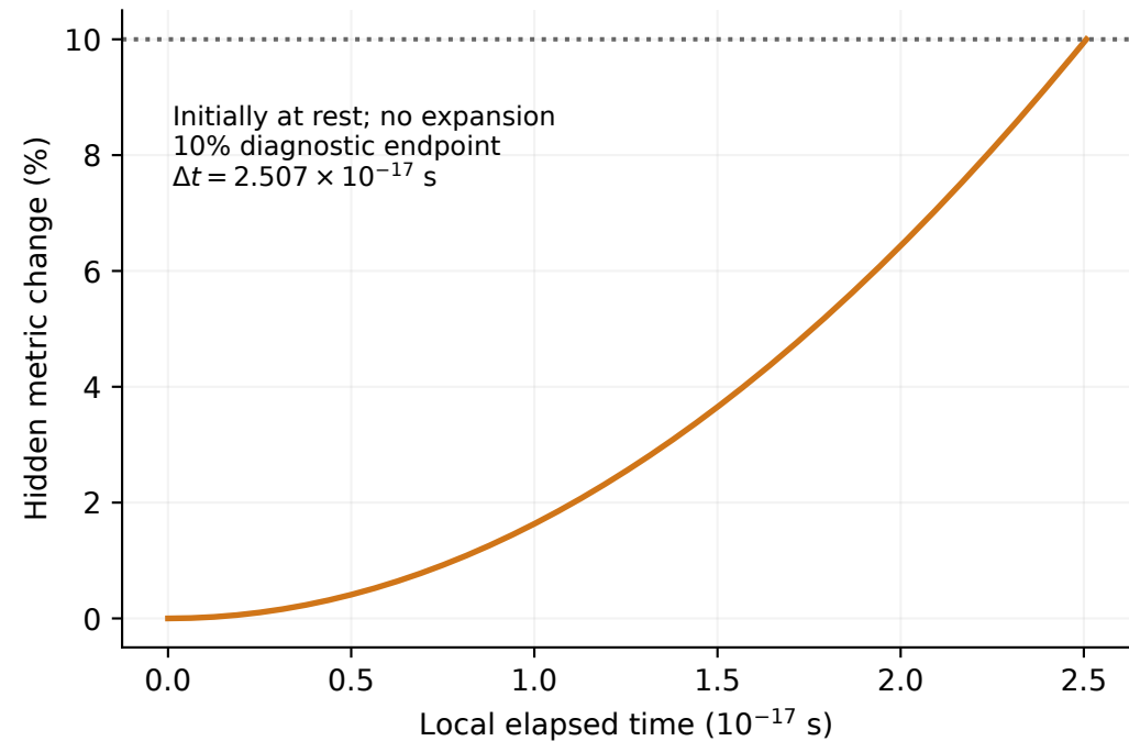
(d) Fixed-source Minkowski transient
