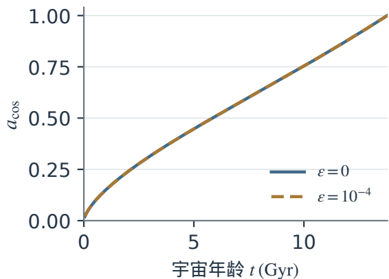
(d) a=0.1 , z=9 t=0.542 Gyr
