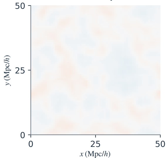
(d) a=0.1 , z=9 t=0.542 Gyr
