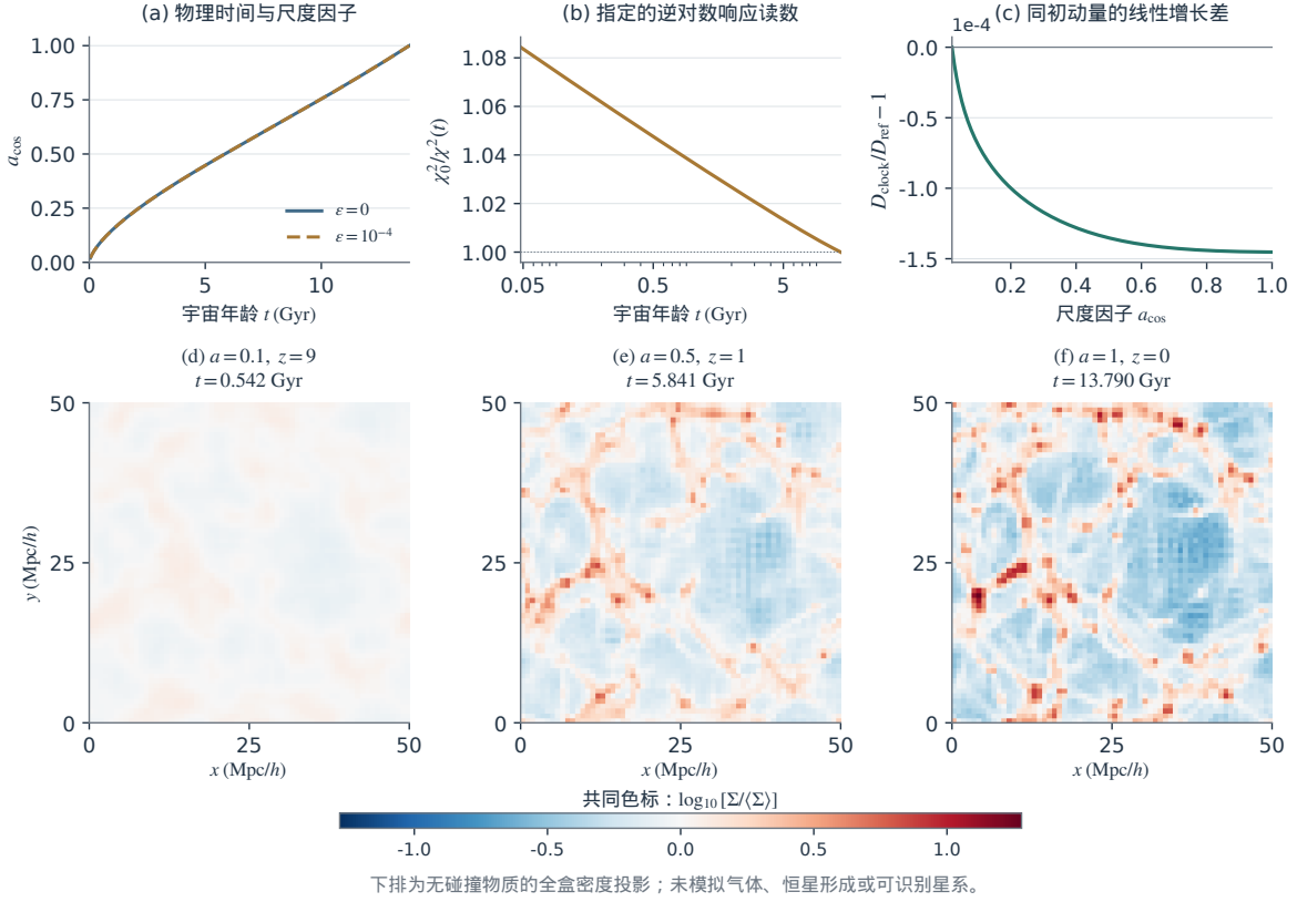
图4.4 从物理背景到无碰撞物质聚类。 上排为尺度因子与年龄、时钟归一化响应 \chi_0^2/\chi^2 及相同初动量下的线性增长差；下排为主例在 z = 9, 1, 0 的实际存档密度投影，使用共同对数色标。标准引力及外部CAMB初谱是本轮的物理输入，两背景共享同一初态。主格距 0.78125 \text{ Mpc}/h 、每粒子质量 4.17 \times 10^{10} M_\odot/h ；本图展示物质聚类，未分辨星系。功率图、各分辨率结果及核验见实验归档。 57
