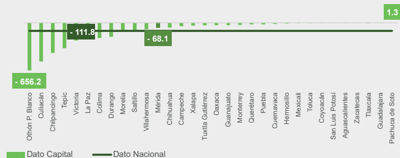
Gráfica 4. Emisiones netas de carbono por ciudad capital
