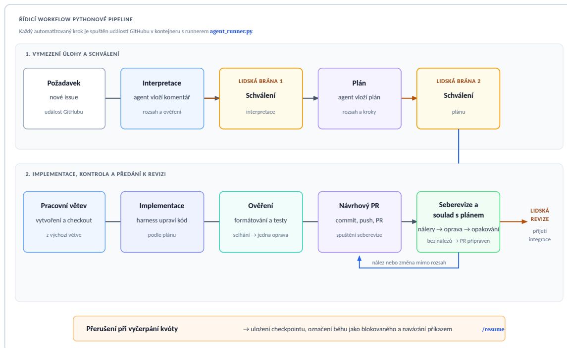
Obrázek 4: Řídící workflow Pythonové pipeline DarkFactory. Schéma zachycuje průchod od nového požadavku přes dvě schvalovací brány, implementaci a opakovanou seberevizu až po lidskou revizi pull requestu; větev přerušení odpovídá zachování checkpointu a obnovení běhu (26) .
