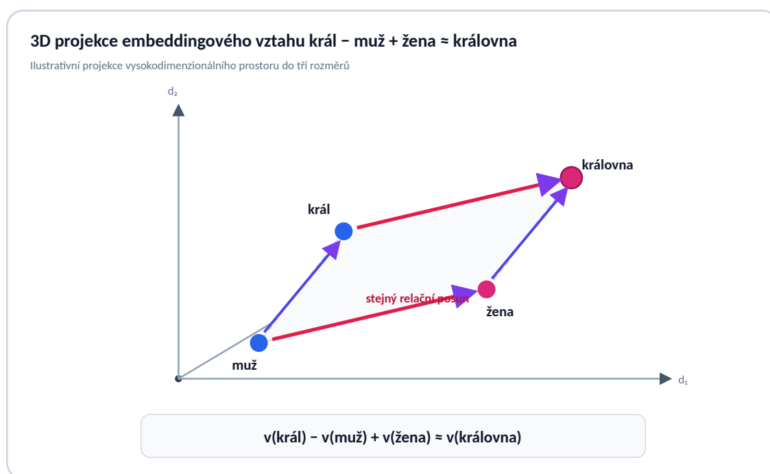
Obrázek 6: Třírozměrná projekce příkladu vektorového vztahu král - muž + žena ≈ královna. Embedding propojuje diskrétní vstupy s numerickým prostorem, v němž lze některé vztahy mezi reprezentacemi vyjádřit směrem a vzdáleností vektorů.
