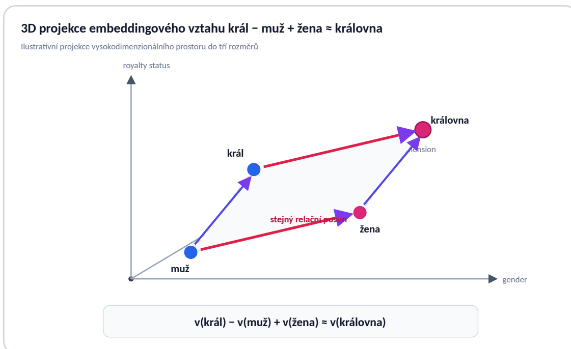
Obrázek 3: Třírozměrná projekce příkladu vektorového vztahu \text{král} - \text{muž} + \text{žena} \approx \text{královna} .
