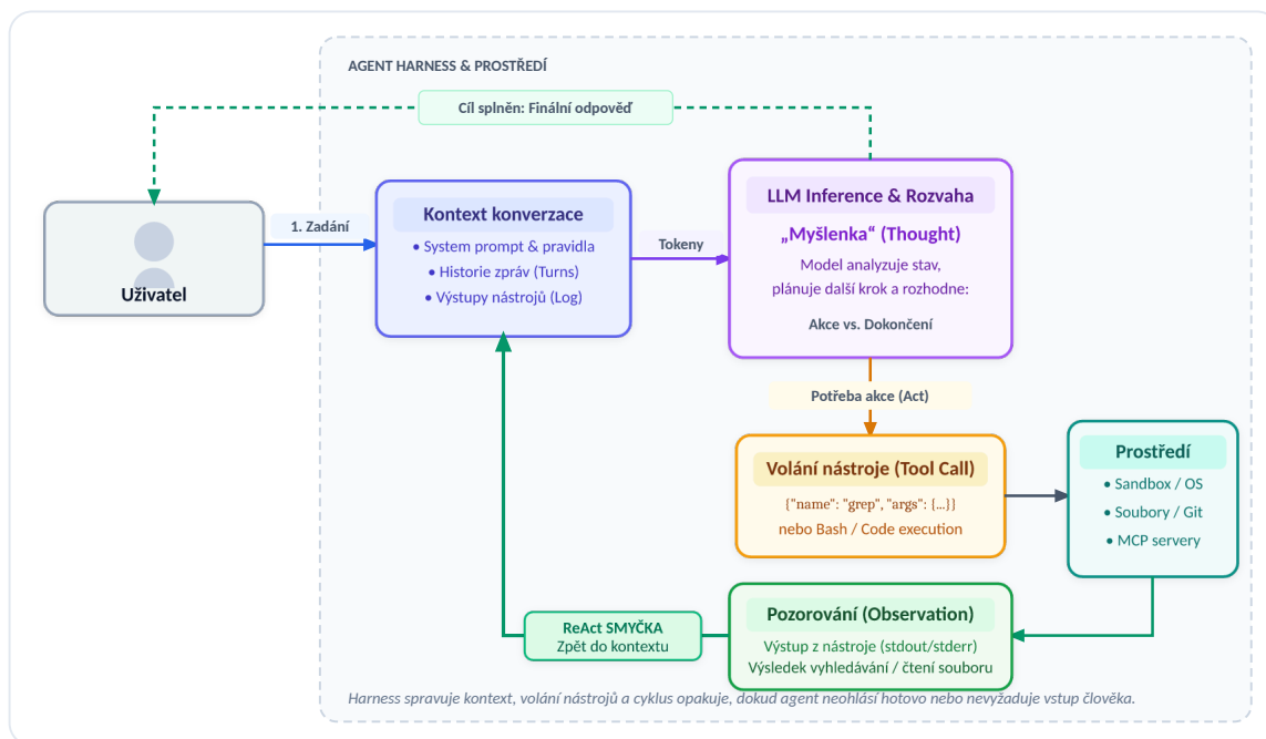
Obrázek 9: Architektura autonomní ReAct smyčky a tok dat mezi uživatelem, kontextem, modelem a výkonným prostředím.
