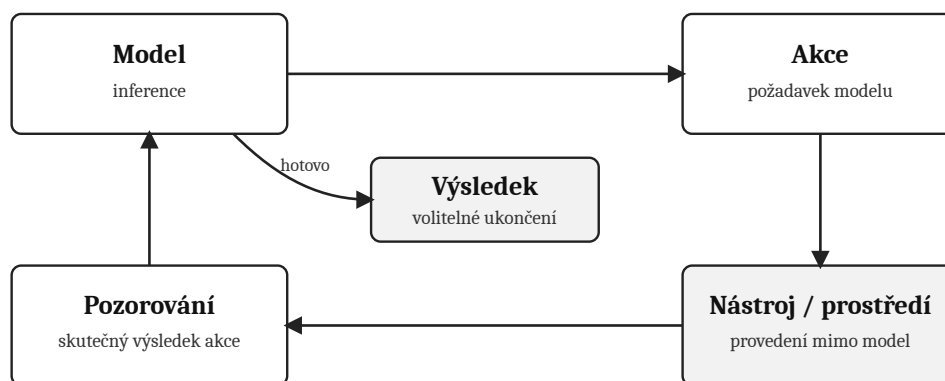
Obrázek 8: Schéma agentní smyčky inspirované interakcí ReAct: model volí akci, Harness ji předá nástroji nebo prostředí, pozorování výsledku se vrací modelu a cyklus může skončit výsledkem. ReAct je zde zdrojem mechanismu, nikoli tvrzením, že každý agentní systém používá totožnou architekturu. (29)
