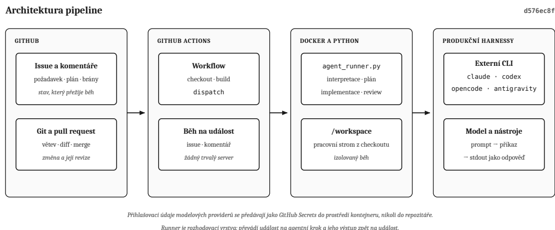
Obrázek 11 — Architektura DarkFactory (35).
