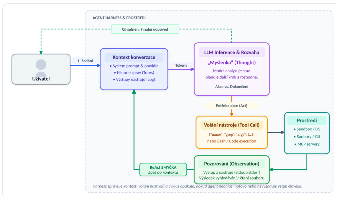
Obrázek 10: Architektura autonomní ReAct smyčky a tok dat mezi uživatelem, kontextem, modelem a výkoným prostředím.
