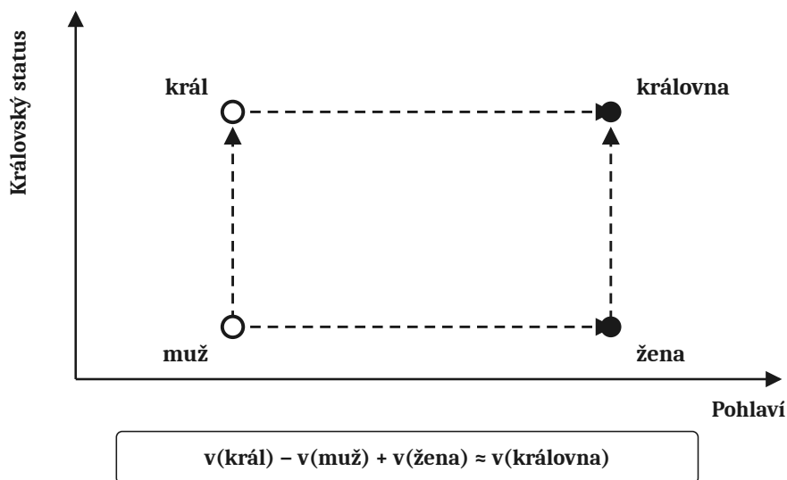
Obrázek 2: Ilustrace sémantického vztahu mezi vektorovými reprezentacemi slov král , královna , muž a žena (29).
