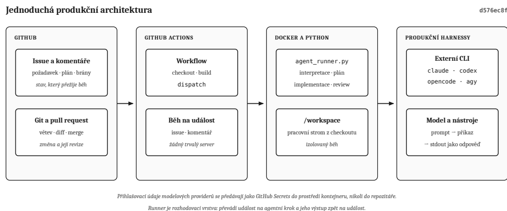
Obrázek 4: Architektura: GitHub poskytuje události a vývojový stav, GitHub Actions výpočet, Docker odděluje běh a pythonovský runner převádí událost na agentní krok. Produkční harnessy claude , codex , opencode a agy zajišťují model, nástroje a pozorování (35).
