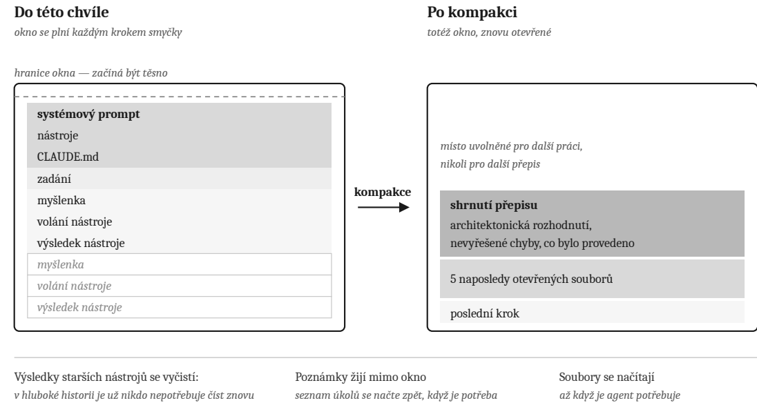
Obrázek 6: Kontextové okno v Claude Code: systémový prompt, nástroje a zadání zůstávají, zatímco myšlenky, volání nástrojů a jejich výsledky se vrší. Když okno dojde k hranici, kompakce nahradí přepis souhrnem a běh pokračuje s ním a s pěti naposledy otevřenými soubory. Vedle toho běží tři věci: výsledky starších nástrojů se čistí, poznámky se ukládají mimo okno a obsah souborů se načítá až tehdy, když je agent potřebuje (20).
