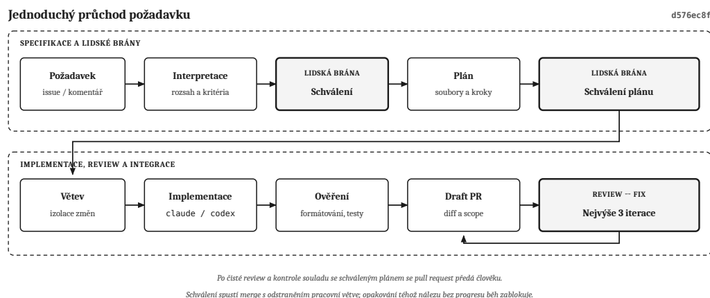
Obrázek 6: Průchod požadavku: implementace a plánování jsou odděleny lidskými bránami, implementace probíhá na větvi a review smyčka se opakuje, dokud nálezu nezmizí, v této revizi nejvýše třikrát (26).
