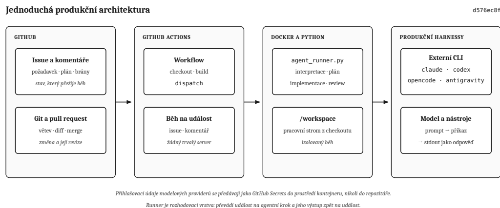
Obrázek 5: Architektura: GitHub poskytuje události a vývojový stav, GitHub Actions výpočet, Docker odděluje běh a pythonovský runner převádí událost na agentní krok. Produkční harnessy zajišťují model, nástroje a pozorování; registr jich má osm, obrázek ukazuje čtyři (26).
