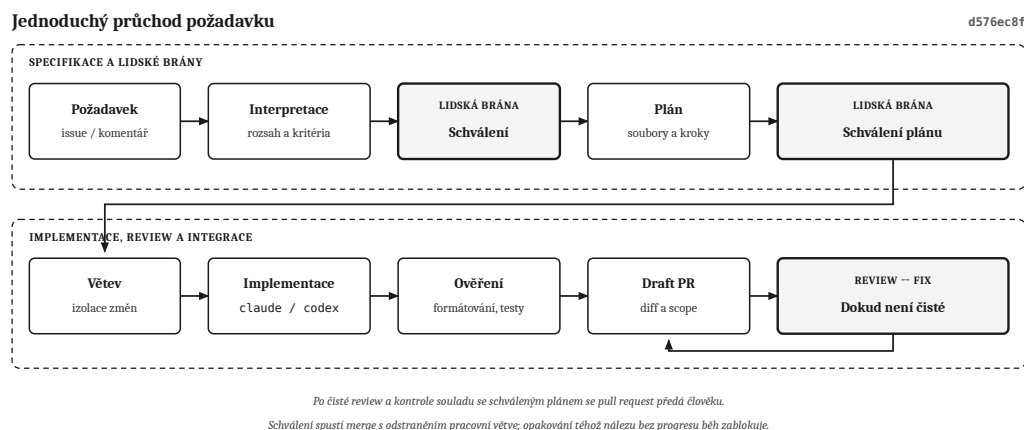
Obrázek 6: Průchod požadavku: implementace a plánování jsou odděleny lidskými bránami, implementace probíhá na větvi a review smyčka pokračuje do vyřešení nálezů (26).
