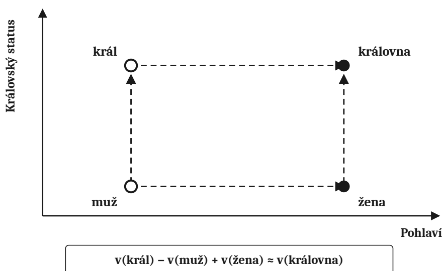
Obrázek 3: Ilustrace sémantického vztahu mezi vektorovými reprezentacemi slov král , královna , muž a žena (30).
