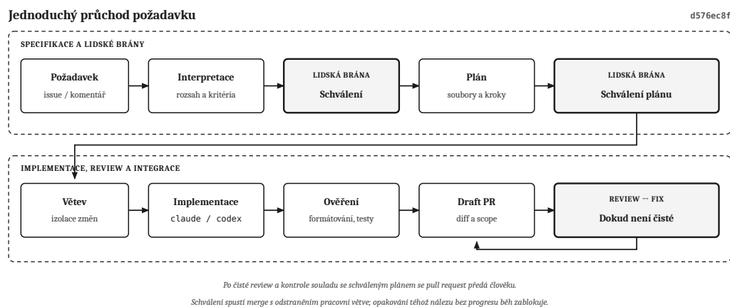
Obrázek 6: Průchod požadavku: implementace a plánování jsou odděleny lidskými bránami, implementace probíhá na větvi a review smyčka pokračuje do vyřešení nálezů (37).
