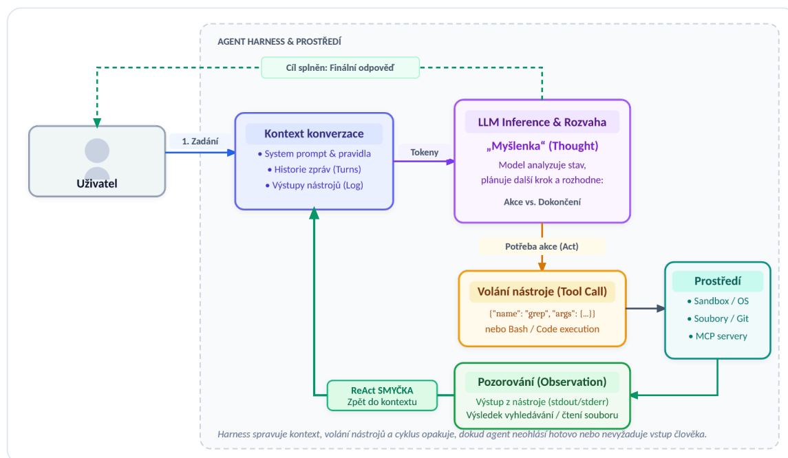
Figure 1: Architektura autonomní ReAct smyčky (Reasoning + Acting) a tok dat mezi uživatelem, kontextem, modelem a výkonným prostředím.
