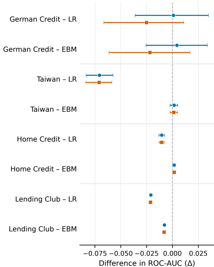
A ROC-AUC
