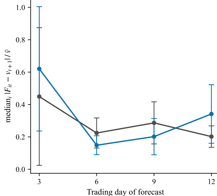
B. Forecast error vs fundamental
