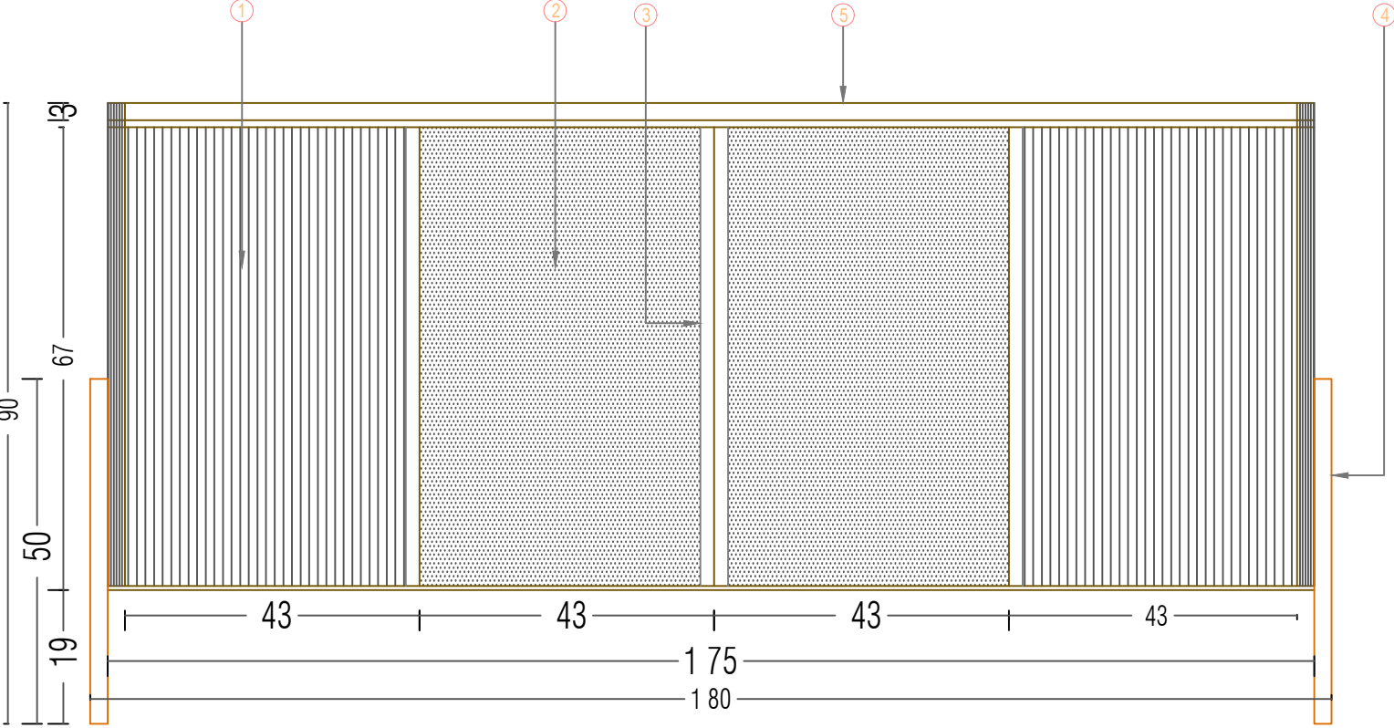
ELEVATION
