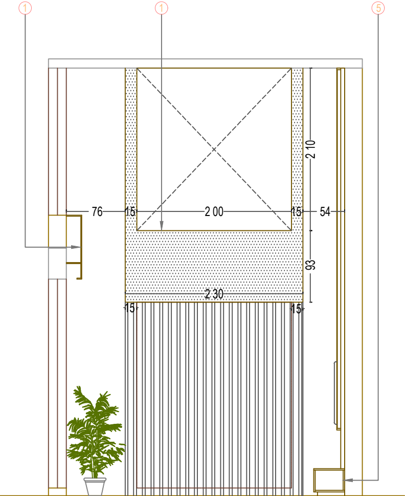
SECTION - DD
