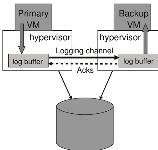
Figure 3: FT日志缓冲区和通道。
