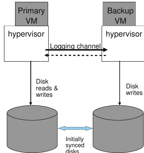
Figure 4: FT非共享磁盘配置。
