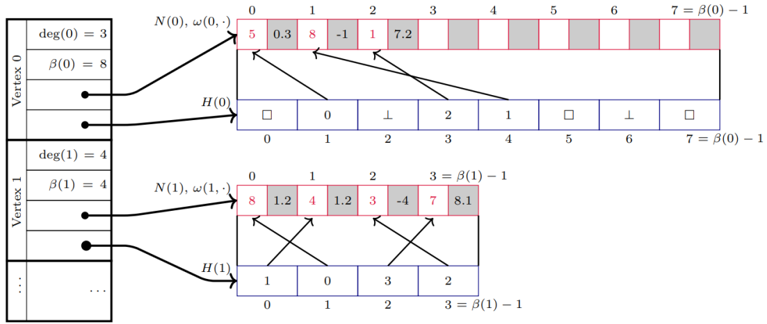
Слика 3.1: Структура хеш-индексираних блокова суседства (DHB) [11]
