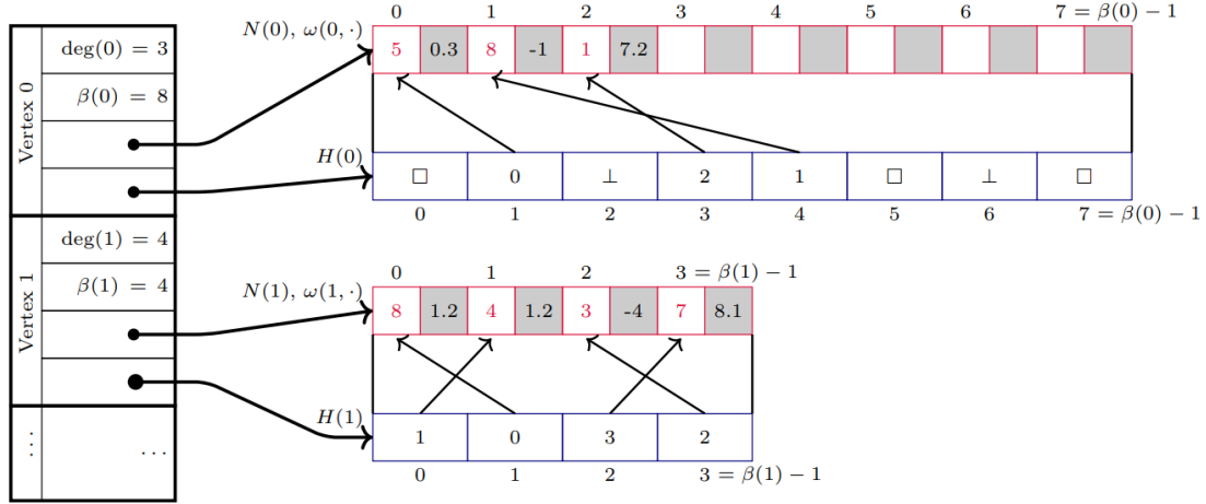
Слика 3.1: Структура хеш-индексираних блокова суседства (DHB) [13]
