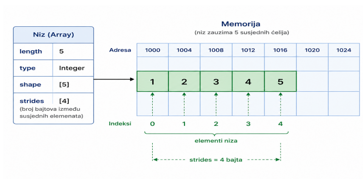
Slika 2.11: Pojednostavljen prikaz memorijske organizacije NumPy niza.
