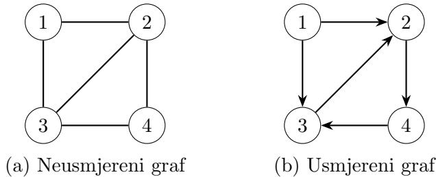
Slika 1.1: Primjeri neusmjerenog i usmjerenog grafa.
