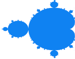
Slika 3.2: MandelbrotoV skup.
