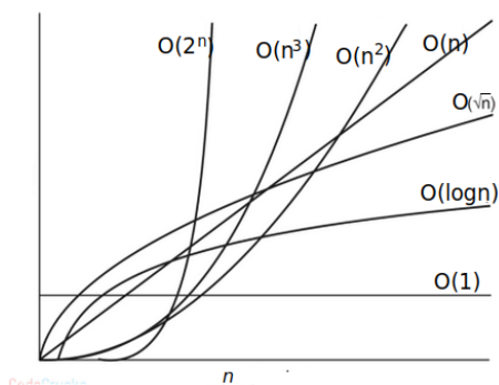
Slika 1.3: Poređenje najčešćih klasa složenosti.
