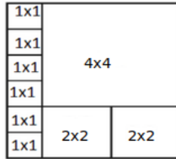
Slika 3.10: Optimalno pokrivanje ploče 6 \times 5
