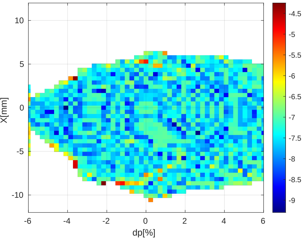
m4Uc-241106-b03-03-09-08 Tune Diffusion Rate
