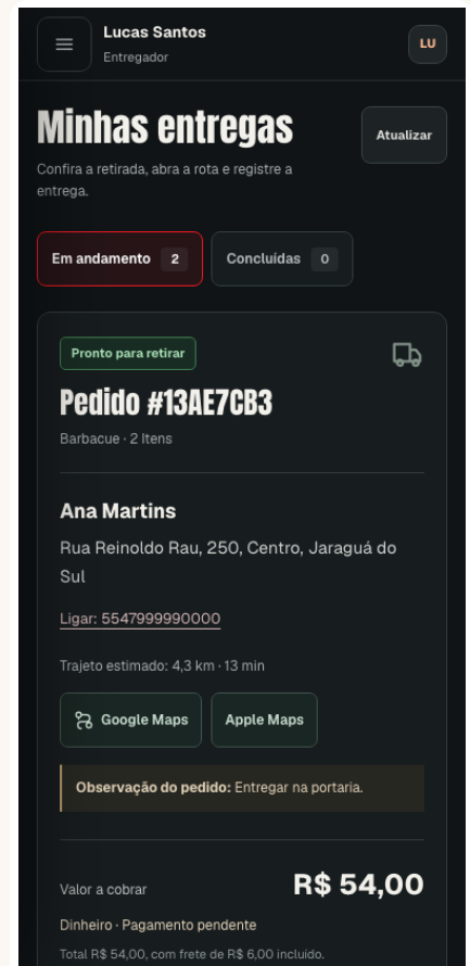
Interface do entregador. Captura de teste com dados ilustrativos.
