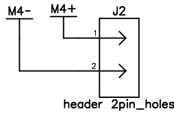
Motor Output
