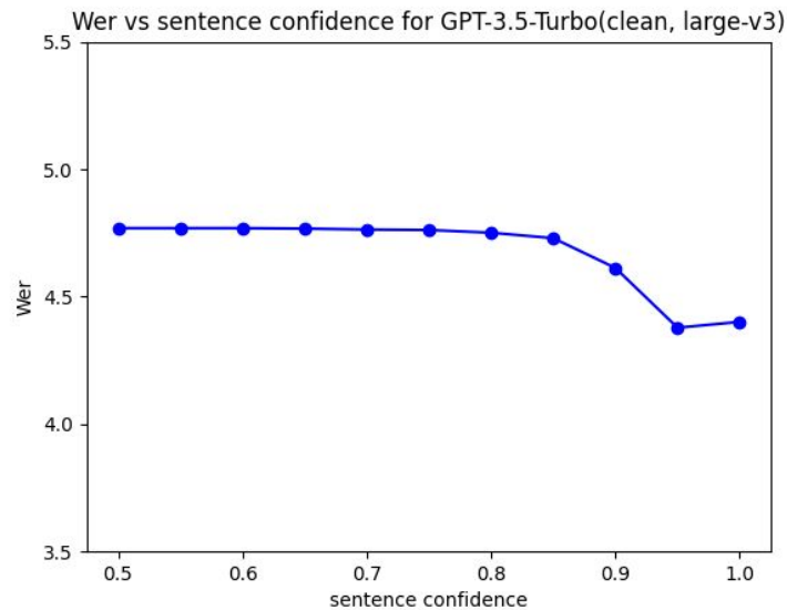
gpt-3.5-turbo-1106
