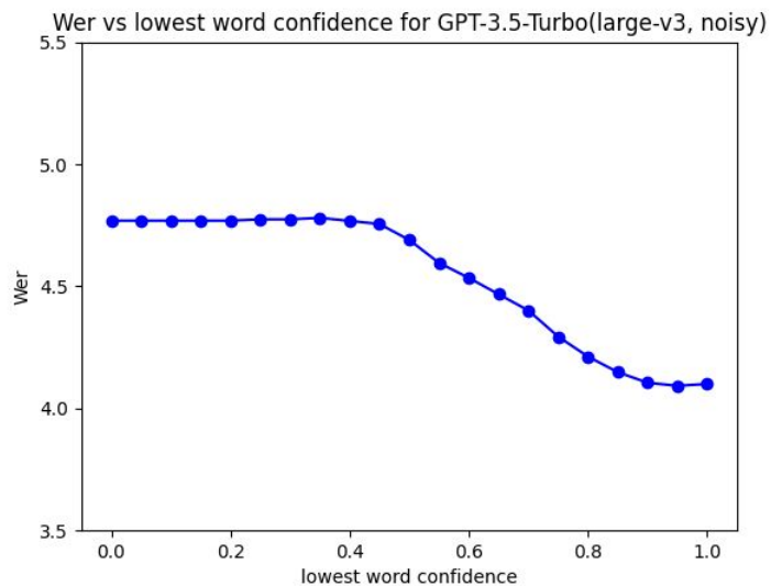
gpt-3.5-turbo-0125
