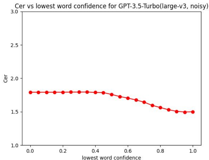
gpt-3.5-turbo-0125
