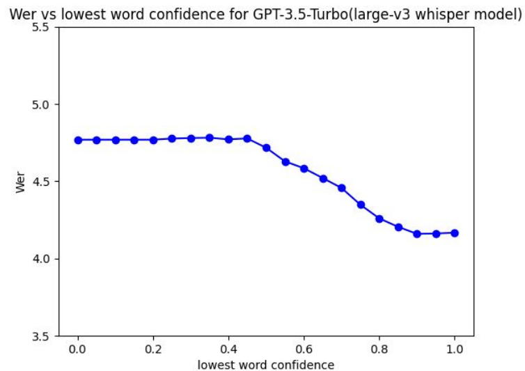
gpt-3.5-turbo-1106
