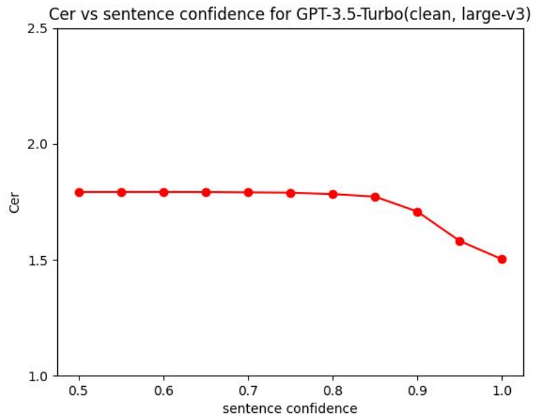
gpt-3.5-turbo-0125
