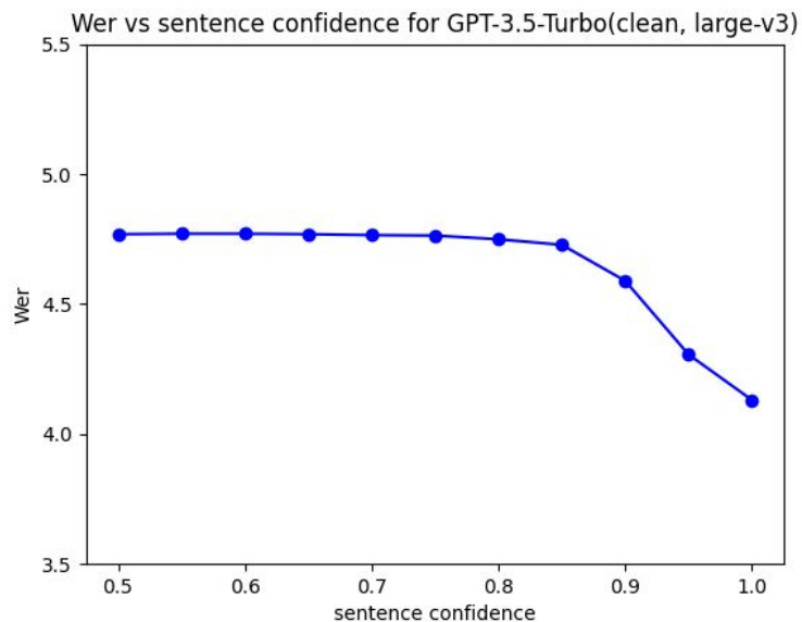
gpt-3.5-turbo-0125
