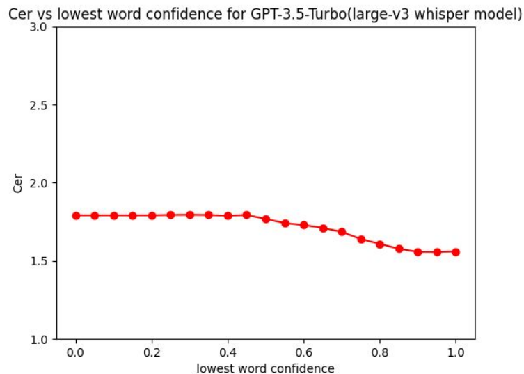
gpt-3.5-turbo-1106
