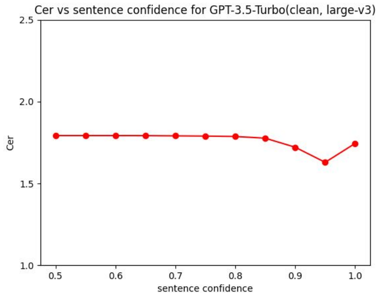
gpt-3.5-turbo-1106
