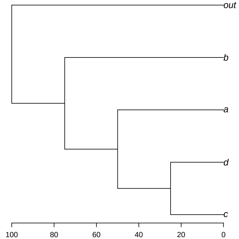
Chronogram
