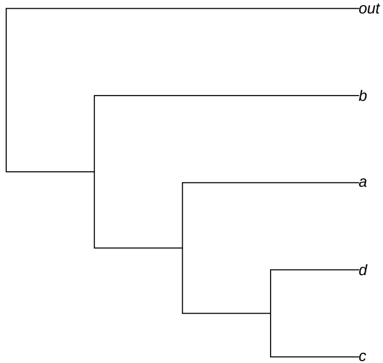
Cladogram
