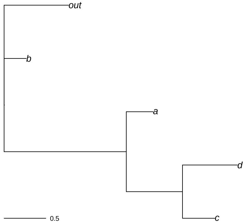
Phylogram
