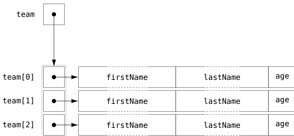
Abbildung 19.1.: Darstellung des Pointers auf ein Array von Pointern auf Player -Objekte
