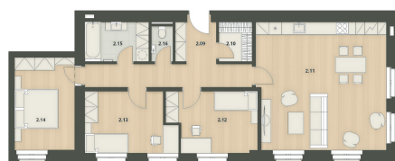
2. nadzemní podlaží
